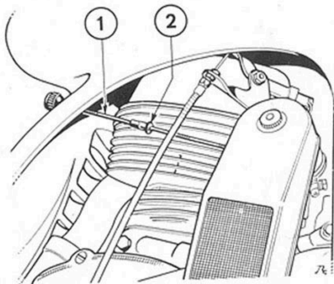
1. Partie de la tige de starter qui reste sur la coque. — 2. Embout fileté SOLIDAIRE DE 1.
