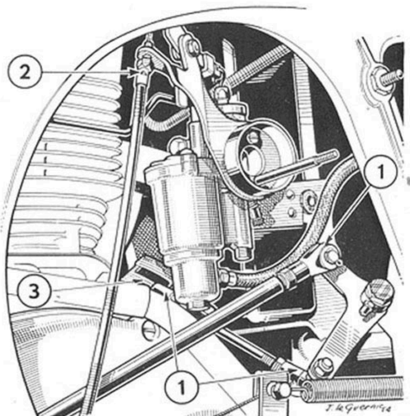
1. Rotules de réglage de tringle de sélecteur — 2. Barillet de réglage de la commande de gaz — 3. Boîtier de sélecteur.
