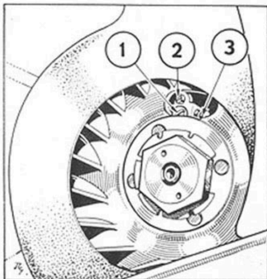
1. Vis de blocage - 2. Vis excentrique de réglage 3. Vis platinées.
