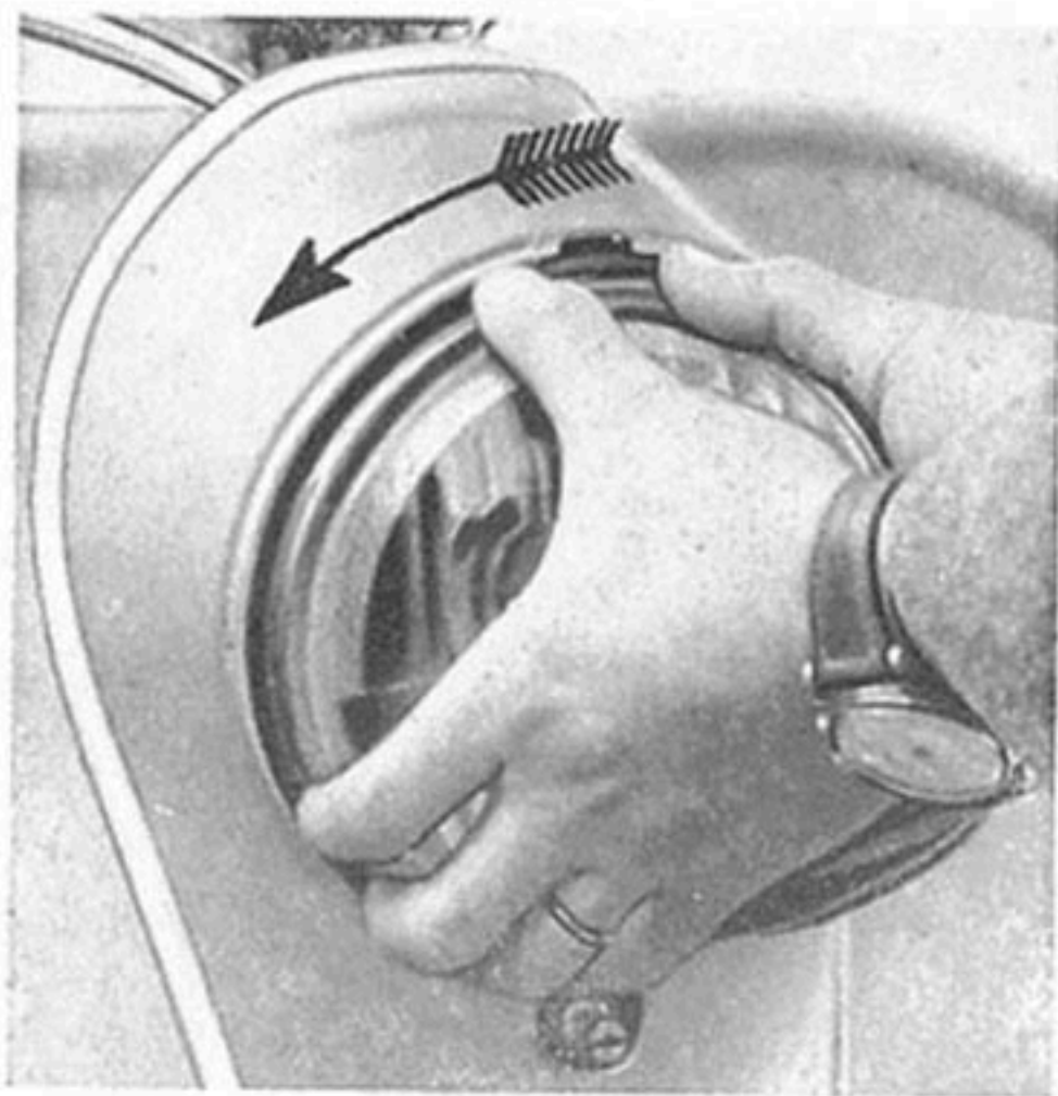
DÉMONTAGE DU PHARE : Appuyer sur le réflecteur et tourner dans le sens de la flèche.
