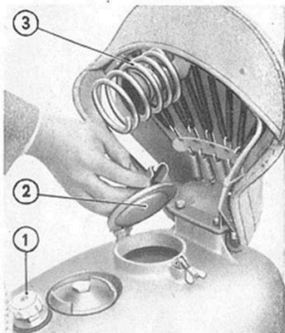
1. Robinet d'essence. — 2. Bouchon du réservoir d'essence. — 3. Pour lever la selle, dévisser le ressort en le tournant vers la gauche.
