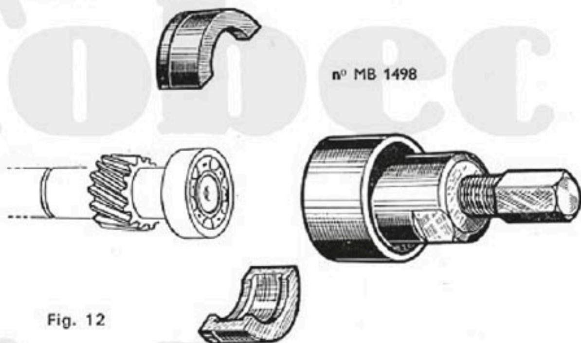
Extraction du roulement 12x28x8 sur arbre primaire
