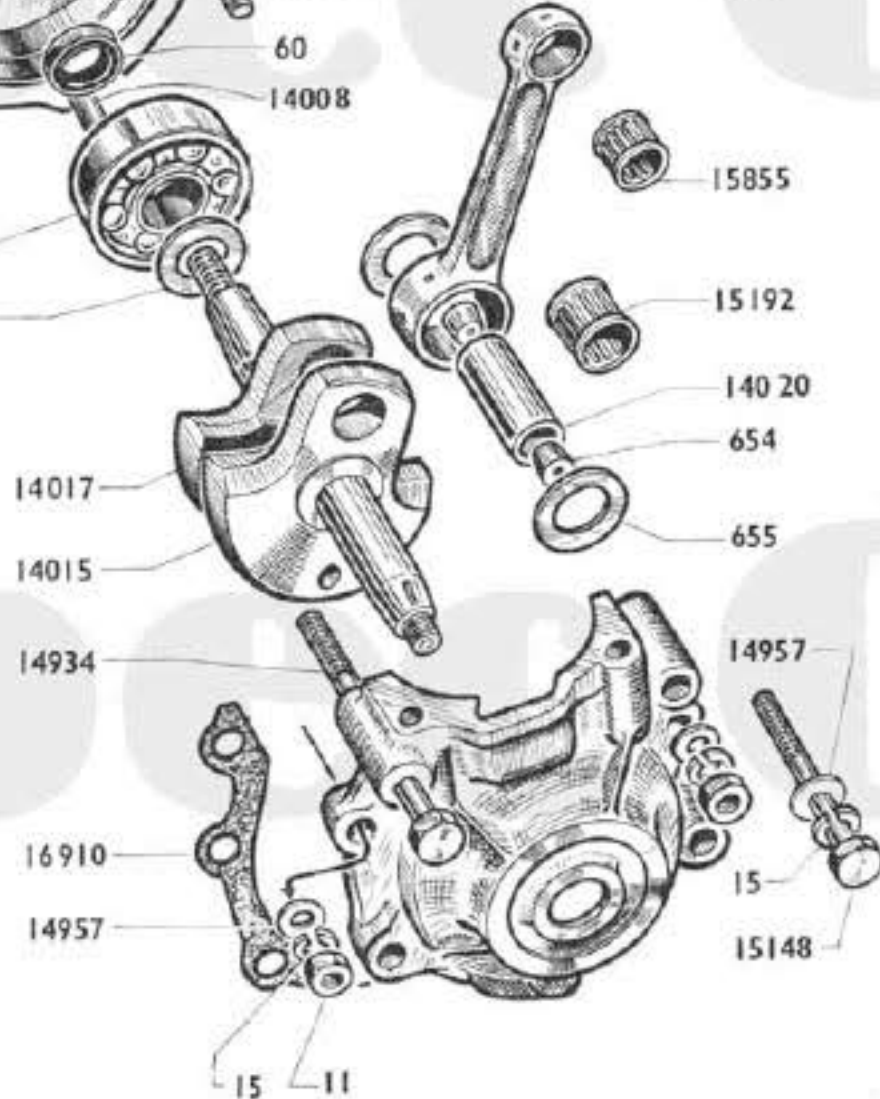
Carter moteur complet 14814
